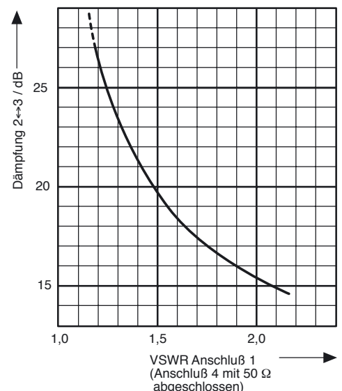
Dämpfung 2↔3 in Abhängigkeit vom VSWR am Anschluß 1
